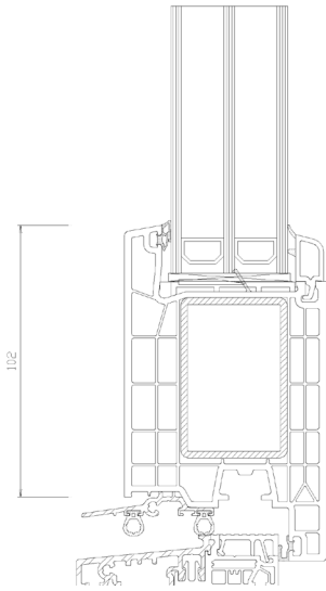
76AD befelé nyíló bejárati ajtó
