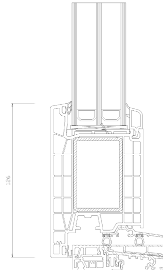
76AD kifelé nyíló bejárati ajtó
